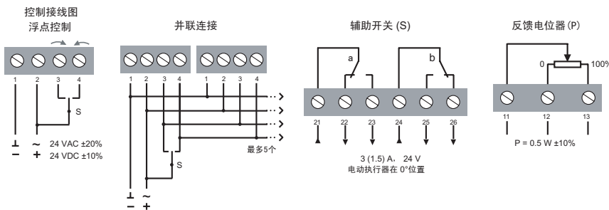
接线图
